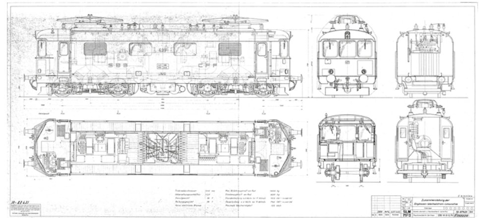
Konstruktionszeichnung Re 4/4 I
