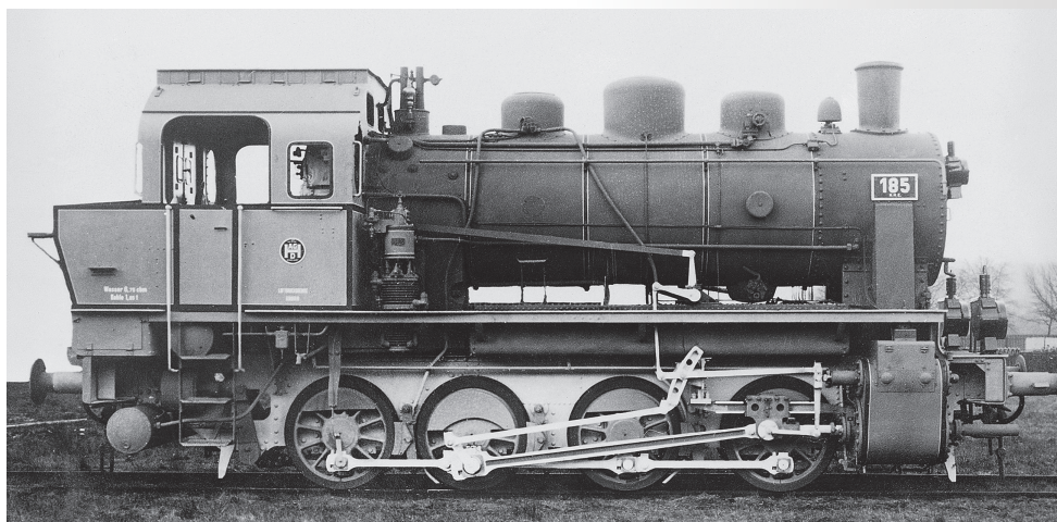
Dampflokomotive Nr. 185 der Halle-Hettstedter Eisenbahn AG Steam locomotive No. 185 of the Halle-Hettstedter Eisenbahn AG
