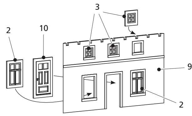
WAND D
