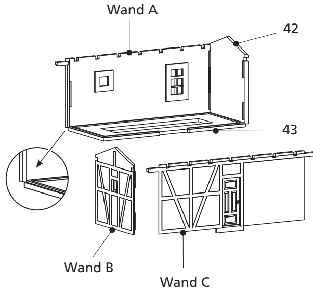
WAND C
