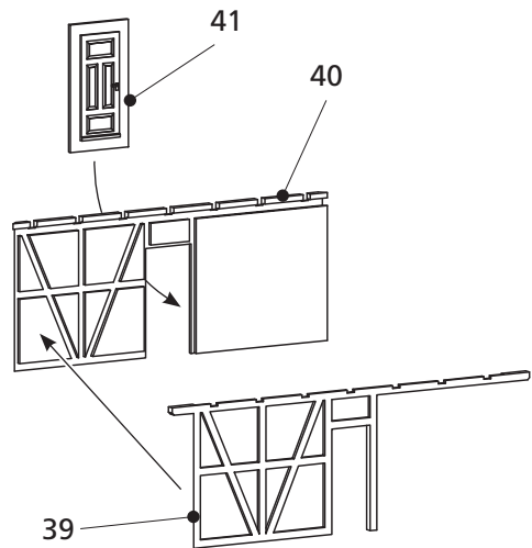
WAND C
