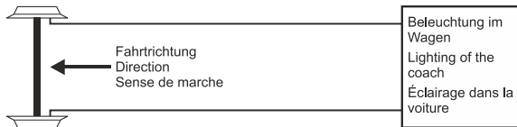
Abb. 3: Prinzipschaltung eines Steuerwagens vor dem Umbau Basic circuit of the control car before conversion Câblage de principe de la voiture-pilote avant installation du décodeur
