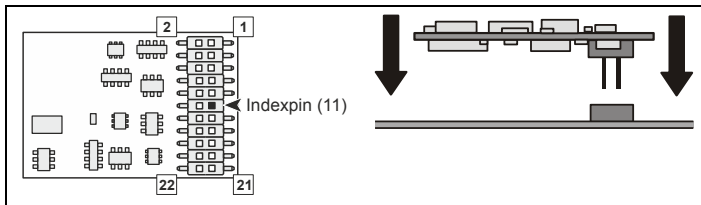
Abb. 1: SILVER+PluX12: 12-polige Schnittstelle /12-pole plug/12-pole Interface
